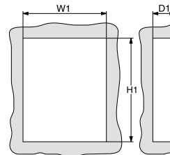
Wymiary dla montażu podtynkowego
