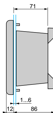
Obudowa wpuszczana GV2-MP (wycięte podłoże)
