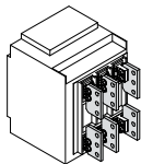
Zaciski wieloprzewodowe dla przewodów miedzianych i aluminium FC CuAl 4x240 mm 2 - FC CuAl
