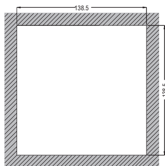
Otwór montażowy
