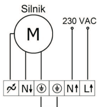
SCHEMAT POŁĄCZEŃ
