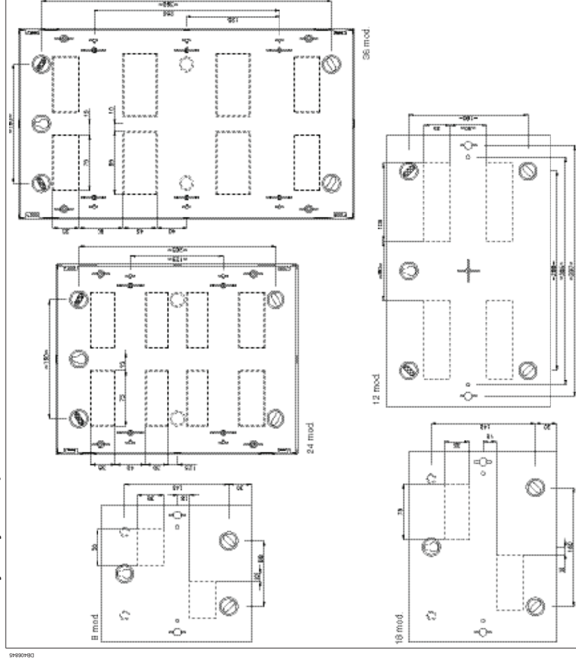
Montaż natynkowy: widok z tyłu
